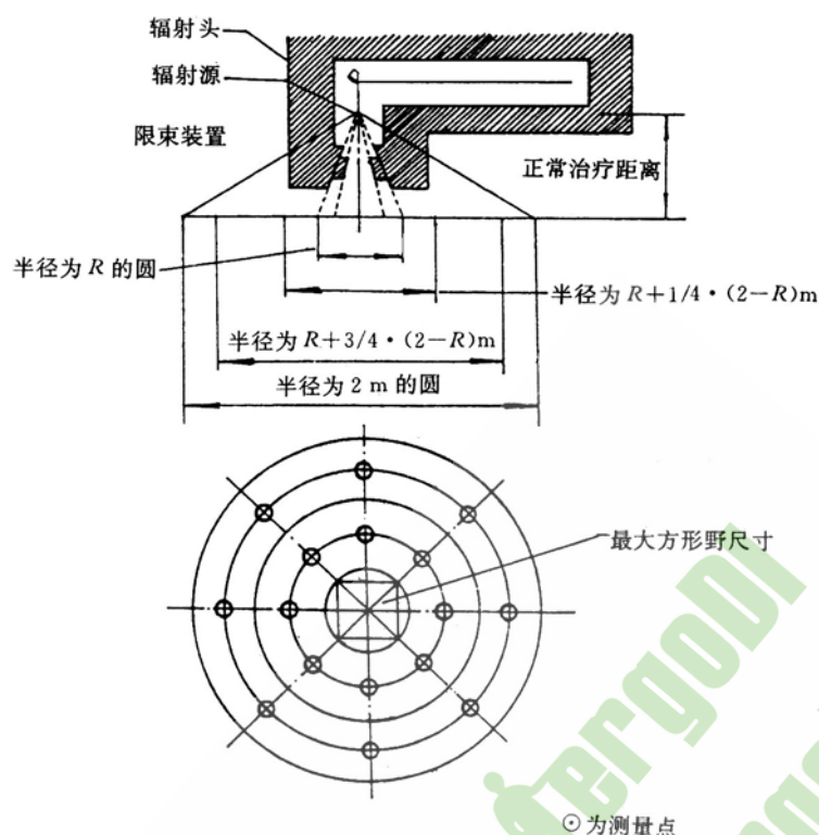
图 A1 平均泄漏辐射 16 个测量点分布
