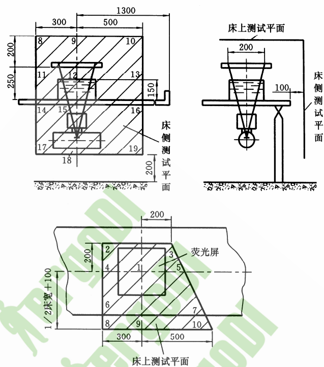
图 A2 卧位透视防护区测试平面示意图 (数字单位: mm)
