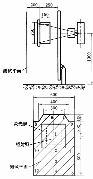
图 A1 立位透视防护区测试平面示意图 (数字单位: mm)
